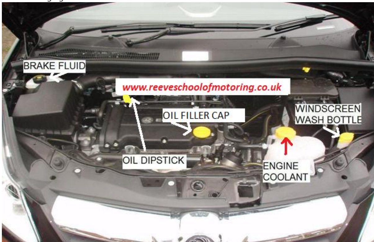
Under the bonnet. Vauxhall Corsa.
